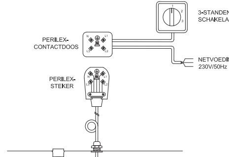
■ Elektrisch aansluitschema perilex
