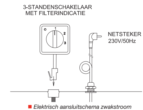
■ Elektrisch aansluitschema zwakstroom
