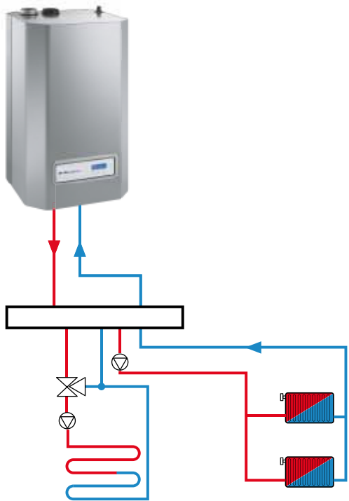
Aansluiting van 2° cv zones op primaire uitgang Combifort2
