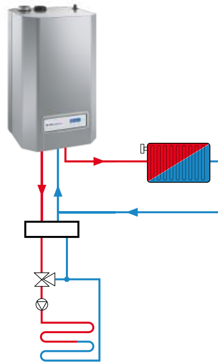
Aansluiting van 1 gemengde cv zone op primaire uitgang Combifort2 samen met aansluiting 2° cv-circuits
