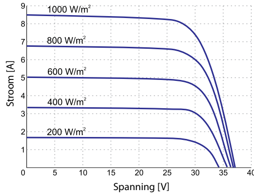
I-V Curve bij Verschillende Zonne-Instralingen
