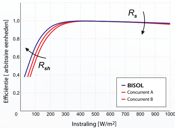
Reële Efficiëntie
