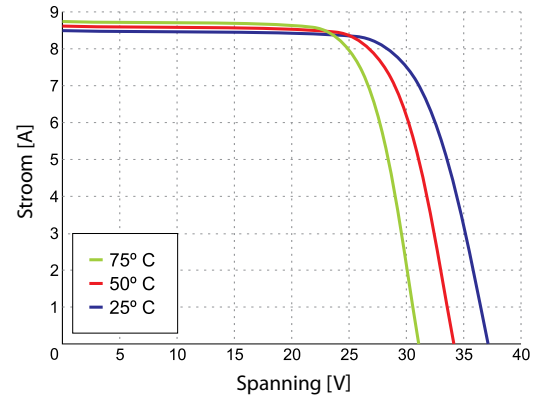
I-V Curve bij Verschillende Celtemperaturen
