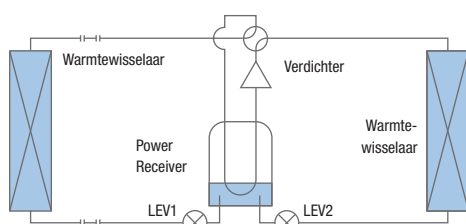
De Power Receiver en de 2 expansieventielen zorgen voor een maximale efficiëntie.
