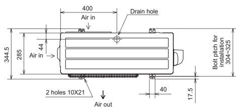
Buitenunits standaard-inverter, SUZ-KA35 VA
