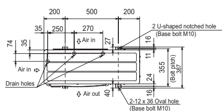
MXZ-4D83/5D102 VA
